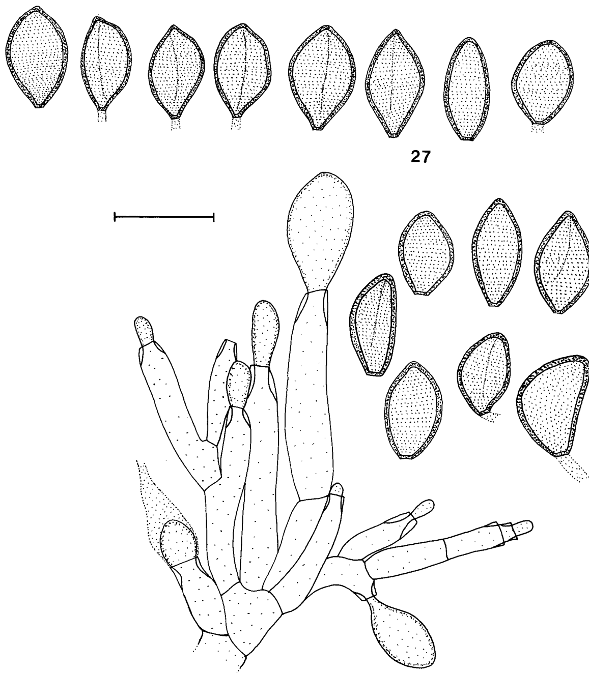
Fig. 27. Conidia and conidiophores of Pilidiella eucalyptorum . Bar = 10 \mu m.
